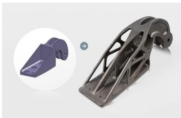
Рисунок 1.14 - Шарнирное крепление до и после оптимизации конструкции под аддитивное производство
