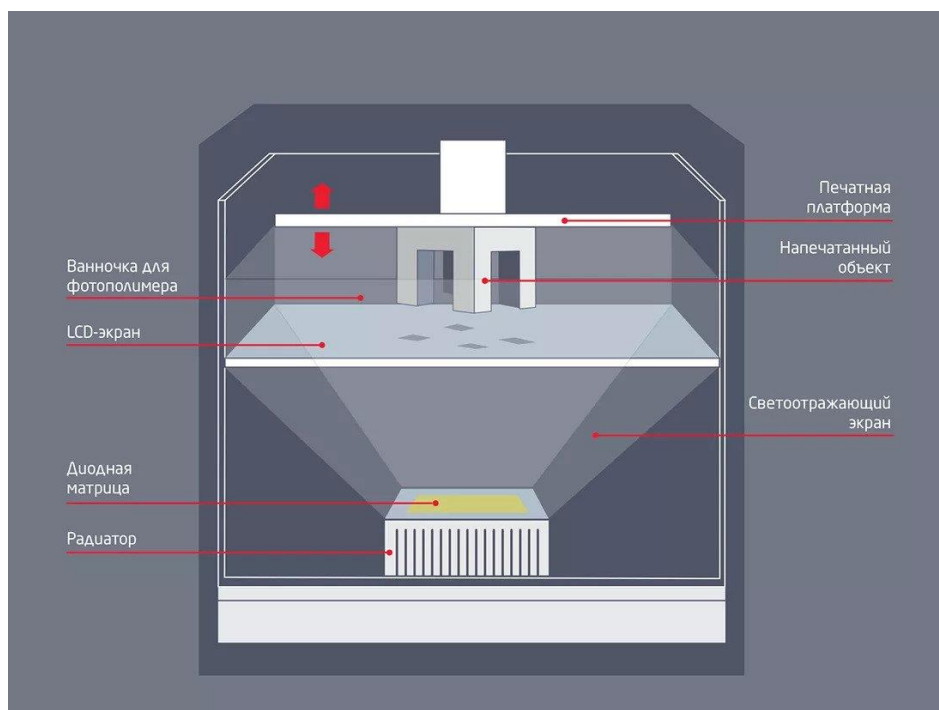
Рисунок 3.4 - Схема LCD-принтера
