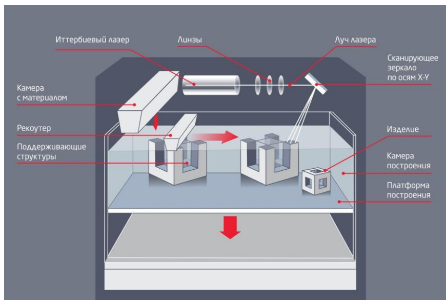
Рисунок 7.2 - Схема SLM-технологии
