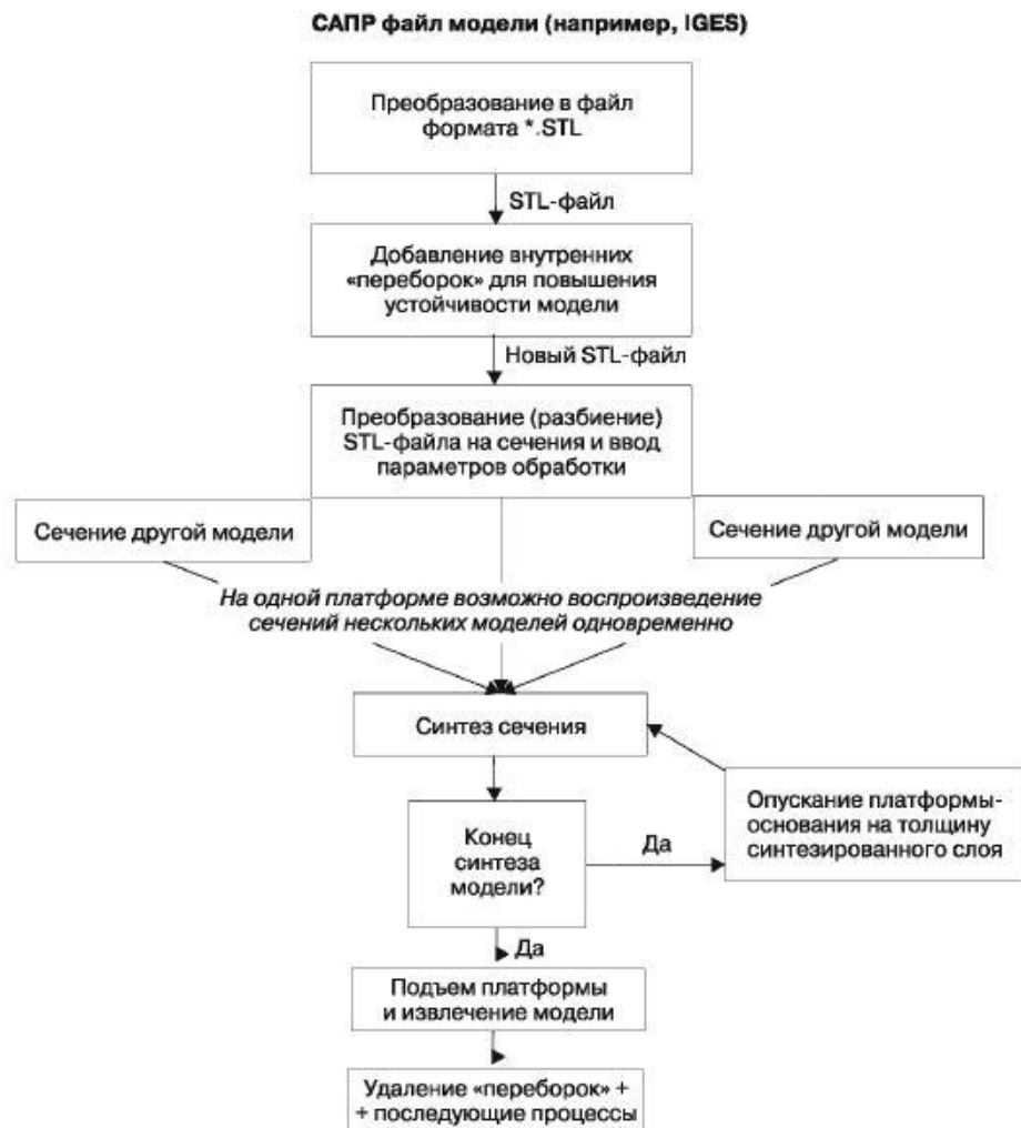
Рисунок 1.8 - Блок-схема управляющей программы обработки с STL-файлом
